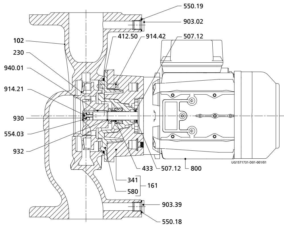
Afb. 7: Overzichtstekening
