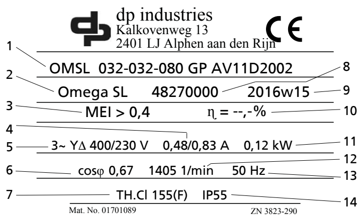
Afb. 2: Typeplaatje (voorbeeld)
