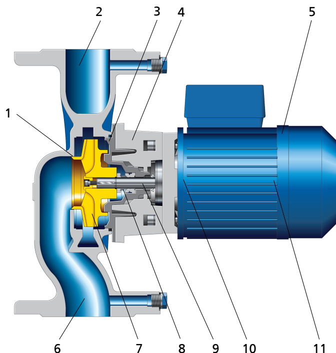
Afb. 3: Doorsnede
